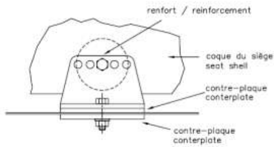
Dessin 253-65 Tekening 253-65
